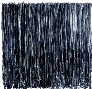
Relief: spelm
